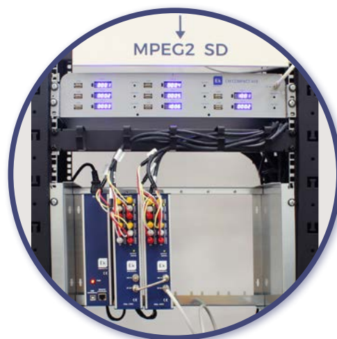
Exemplo do KIT CM COMPACT AV8 instalado num armário rack
