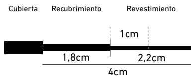
Medidas corte fibra para conector CM SA
