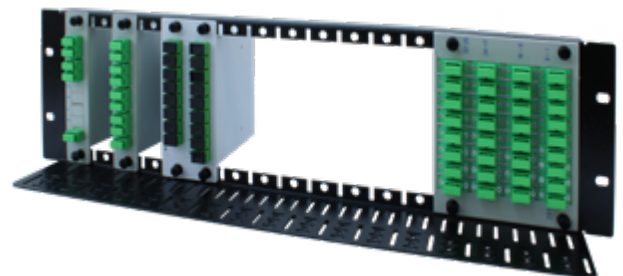
Esempio di splitter SCF montati in un BSCFR
